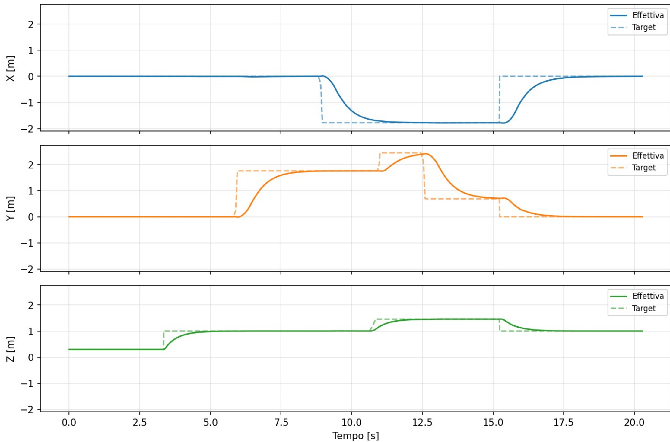
Posizioni vs Tempo — quasi-LPV-MPC (scala comune in metri)
